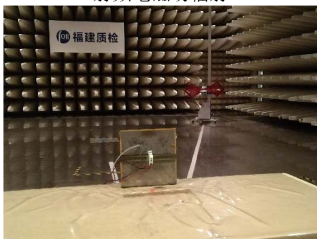
电磁辐射骚扰发射试验
