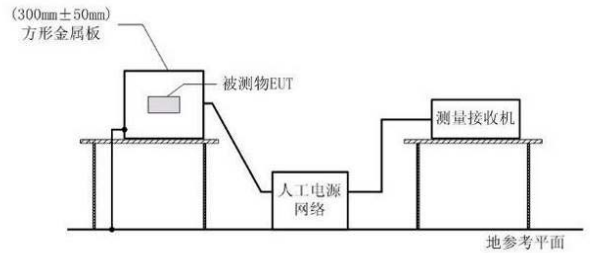
高频发射极限(150kHz 至 30MHz)
