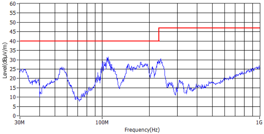
电磁辐射骚扰发射试验预扫描曲线(峰值)
