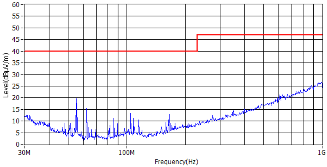
电磁辐射骚扰发射试验预扫描曲线(峰值)
