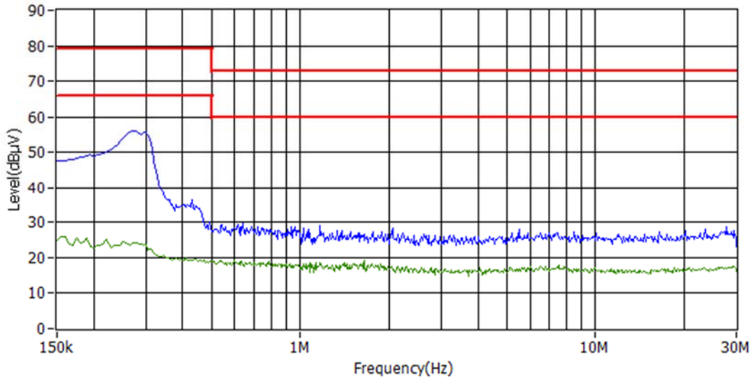
电源端子骚扰发射试验预扫描曲线(峰值)
