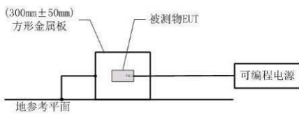
电压暂降和短时中断抗扰度
